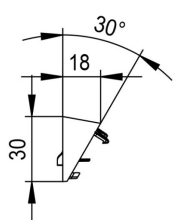
ZUOGN 30° - Seitenansicht
